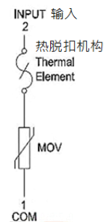
N Type N型式
