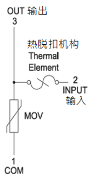
M Type M型式
