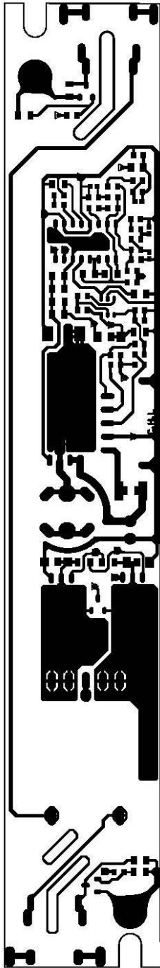
fig-1 Top Layer
